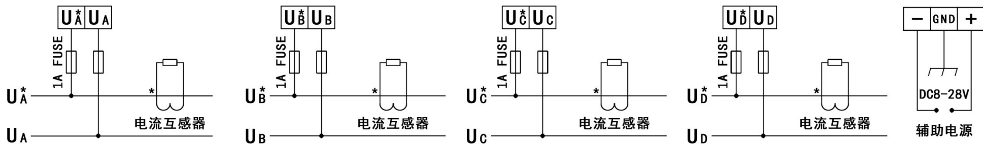
HD450VXXA4TH 四回路交流电流电压采集模块接线图
